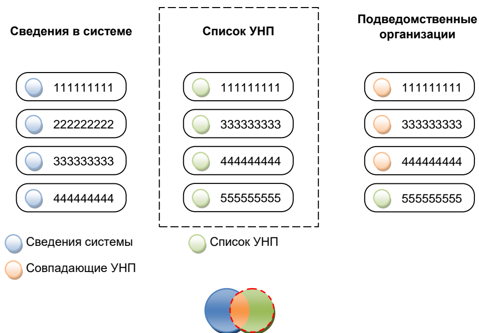
Рис. 5. Формирование списка как единственного источника
